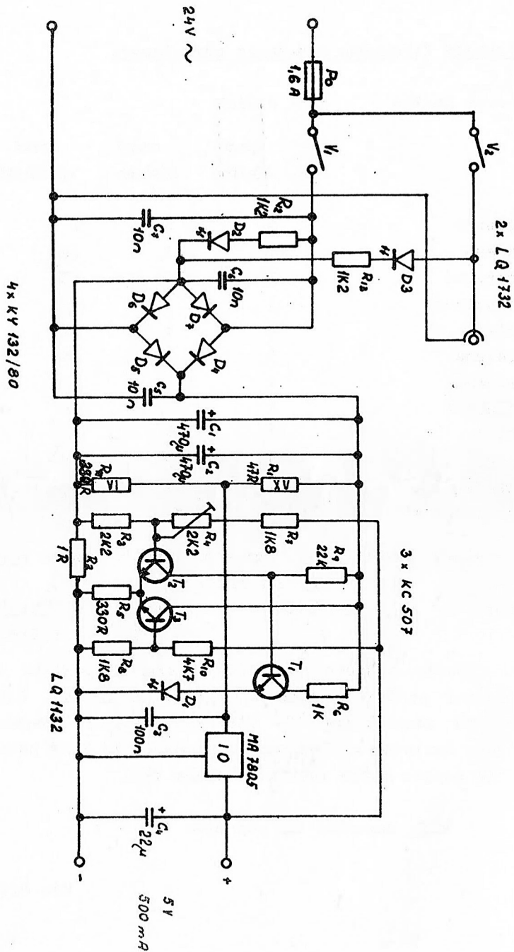
SCHEMA ZAPOJENÍ ZDROJE EES 1
